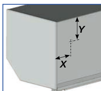
Perçage Ø10mm
